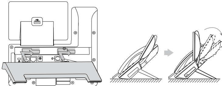
Metodo di montaggio su scrivania
